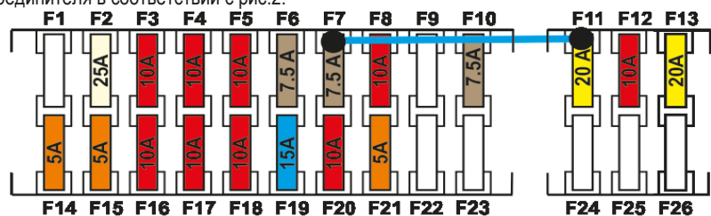
© рис.1 Подключение на автомобиль семейства Лада Приора
