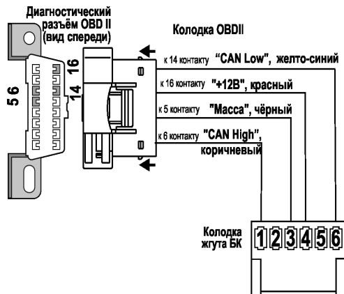
Рис.2 Схема подключения БК "ШТАТ ИСКРА Х1-И"
