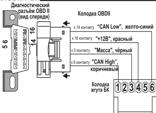
Рис.1 Схема подключения
