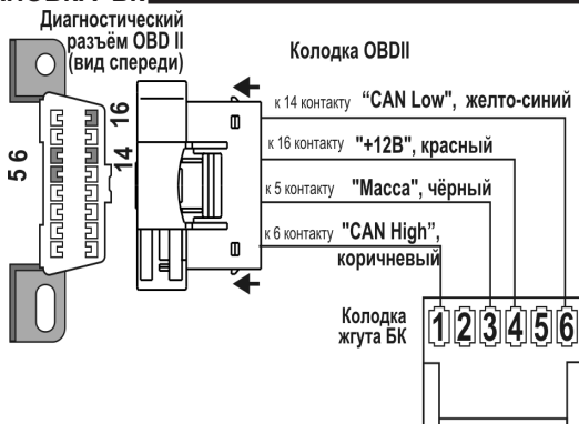
Рис.1 Схема подключения
