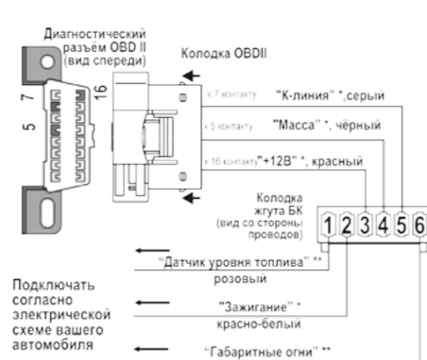
рис.21 Универсальная схема подключения.
