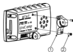
рис.7 Крепление кронштейна к корпусу БК
