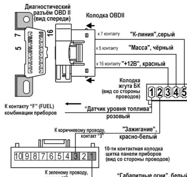
рис.14 Схема подключения к а/м Hyundai Accent с механической коробкой передач
