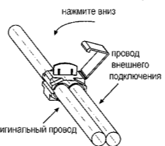
рис.9 Соединение проводов через зажим
