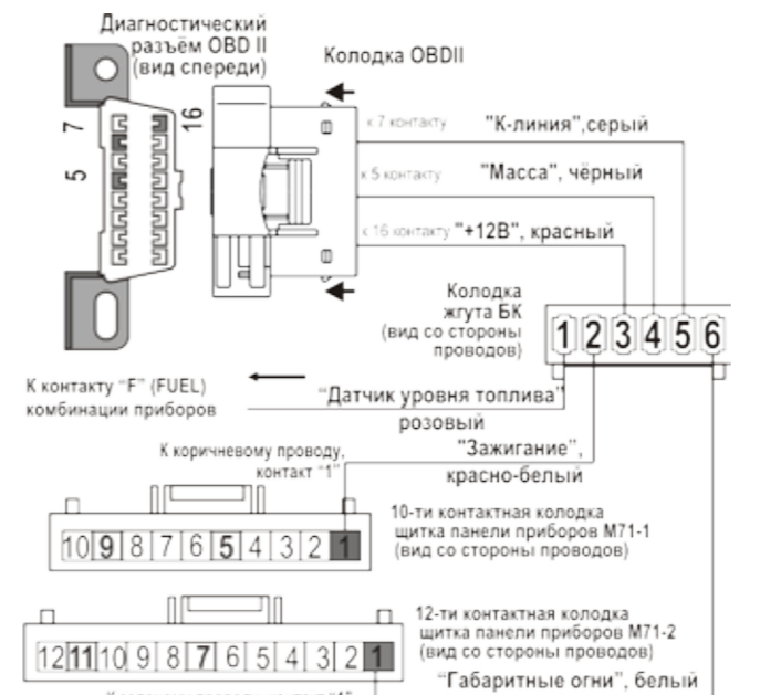
рис.10 Схема подключения к а/м Hyundai Accent с автоматической коробкой передач
