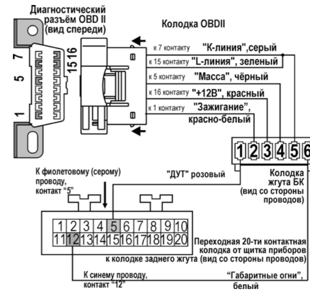
рис.12 Схема подключения Renault Logan
