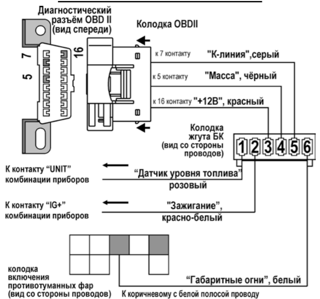
рис.17 Схема подключения к а/м Chevrolet Lanos (после 2008 г.в.) (ЕВРО-3)
