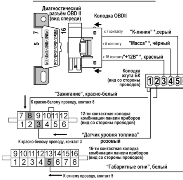
рис.20 Схема подключения к а/м Daewoo Nexia (ЕВРО-3)
