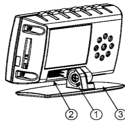
рис.6 Крепление БК на панель приборов
