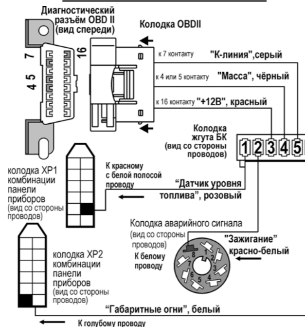
рис.19 Схема подключения к а/м Газель после 2009 г. в. (Микас 10.3)
