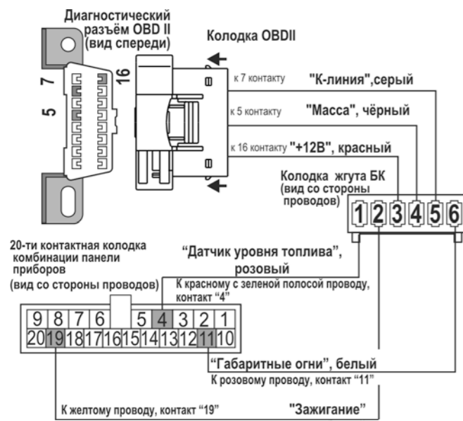
рис.15 Схема подключения к а/м Hyundai Getz (для двух двухрядных колодок комбинации панели приборов)
