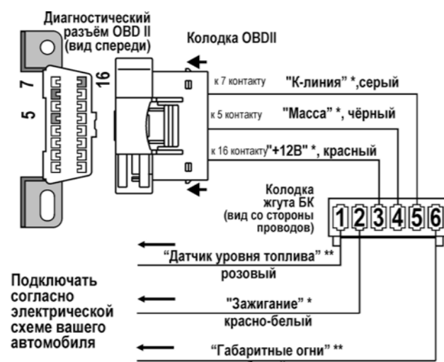
рис.18 Схема подключения к а/м Chevrolet Lacetti и Aveo.
