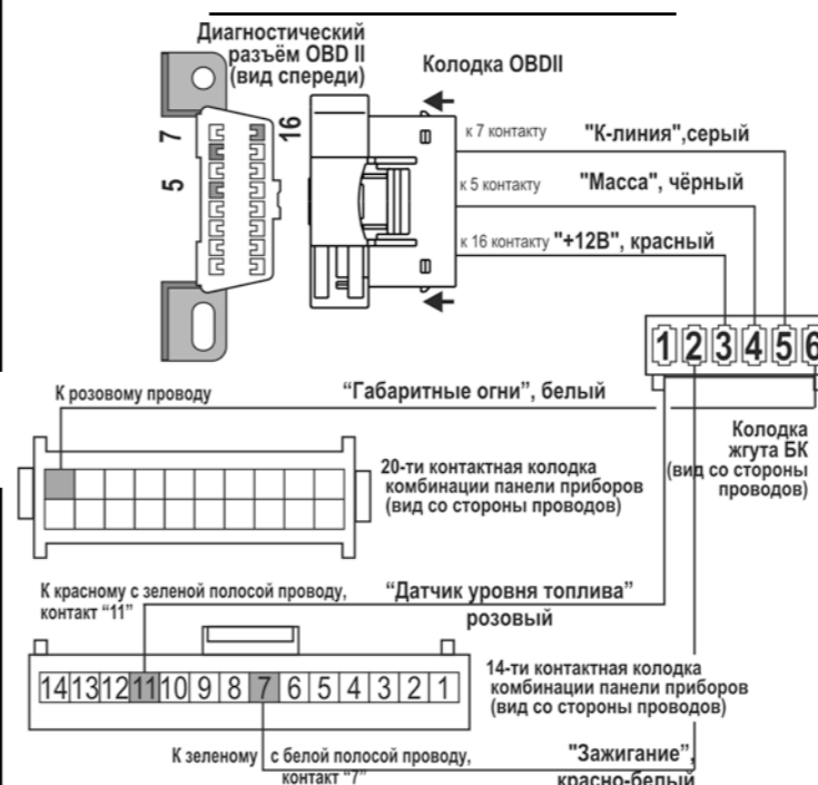
рис.11 Схема подключения к а/м Hyundai Getz (для однорядной и двухрядной колодки комбинации панели приборов)
