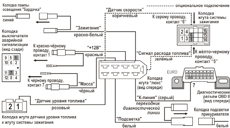
рис.4 Схема подключения (панель "люкс")
