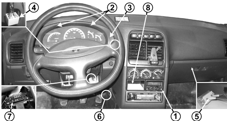
рис. 3 Панель приборов «ЛЮКС»
