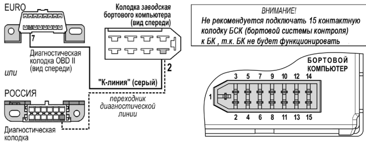
Рис.1 Схема подключения (обычная панель)
